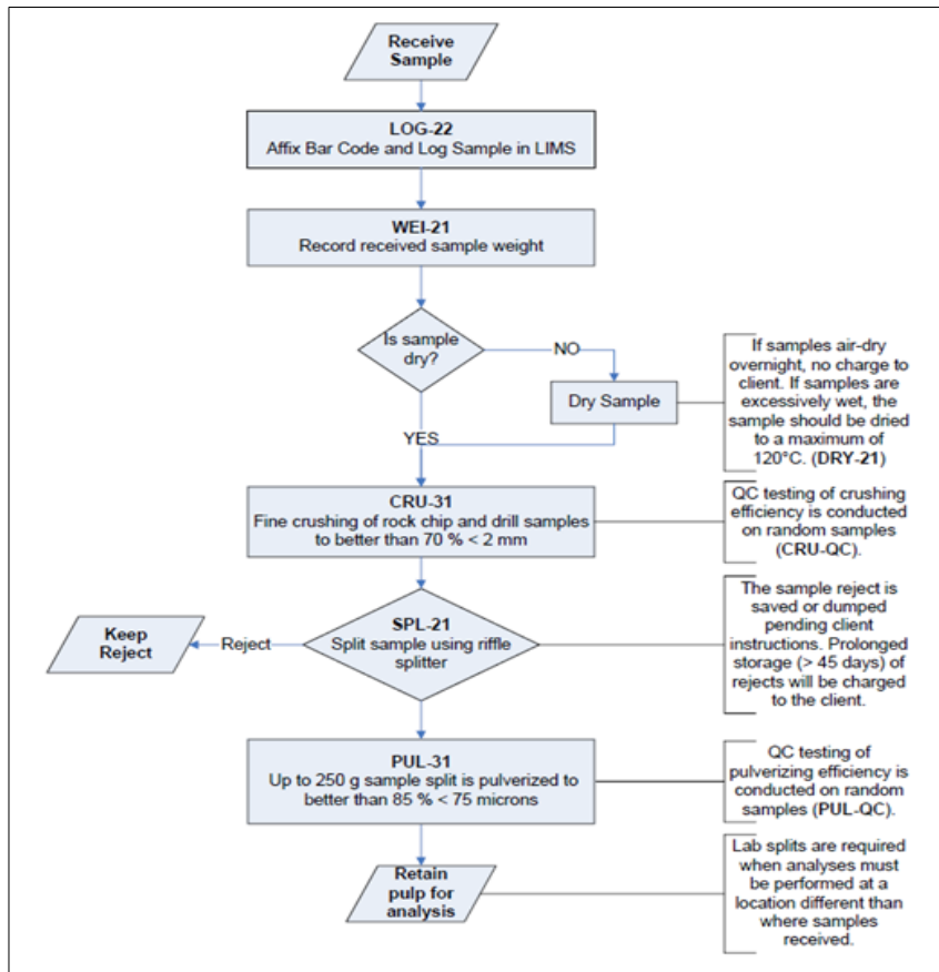
Figure 15: ALS Laboratory Sample Preparation Flow Sheet
